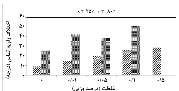
شکل ۱۵- اثر غلظت ذرات نانو بر روی زاویه تماس نانوسیالات با سنگ در دو دمای متفاوت پس از گذشت ۱۵ روز
