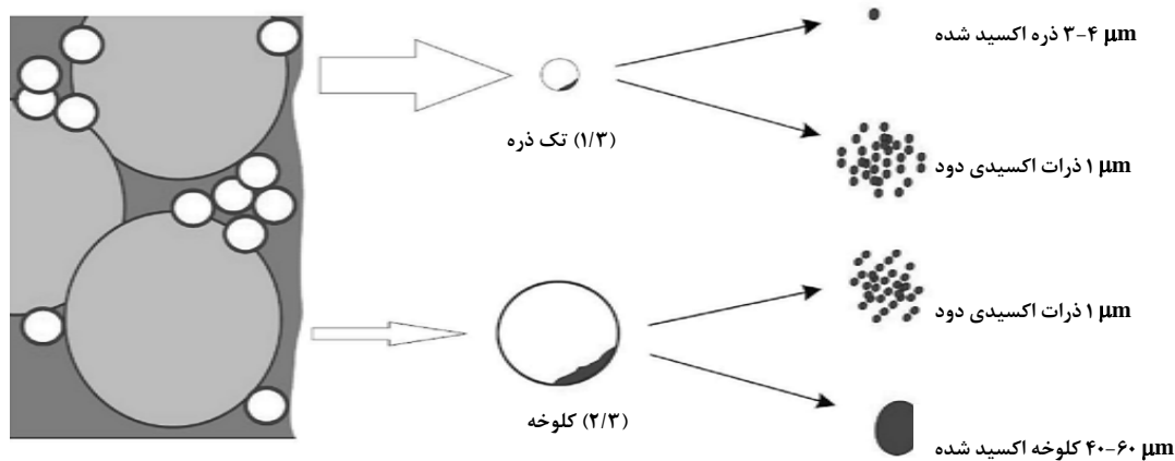
شکل ۳. جدایش ذرات آلومینیم از سطح احتراق پیشراشه‌های جامد چندسازه‌ای [۲۳].
