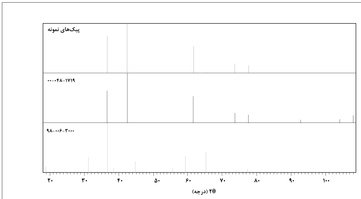
شکل ۴. مقایسه نمودار پیک‌های فازهای نمونه همزهشت شده (منحنی بالا) با پیک‌های استاندارد فازهای
