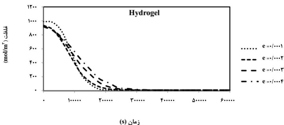
شکل ۶. تأثیر افزایش ضخامت حامل هیدروژل در سرعت رهش ویتامین B12 به‌ازای حرکت مرز با سرعت متغیر.
