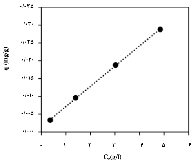
شکل ۱۲. نمودار خطی همدمای لانگمویر برای کربن فعال در دمای ۲۵ درجه سلسیوس (سرعت همزن: ۴۵۰ دور بر دقیقه، مقدار جاذب: ۱ گرم).
