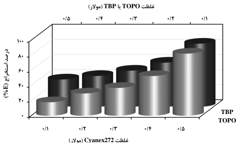
شکل ۳. درصد استخراج کبالت با غلظت‌های متفاوتی از استخراج‌کننده‌های اسیدی در سامانه مخلوط دوتایی Cyanex272 با حلال TOPO و یا TBP.
