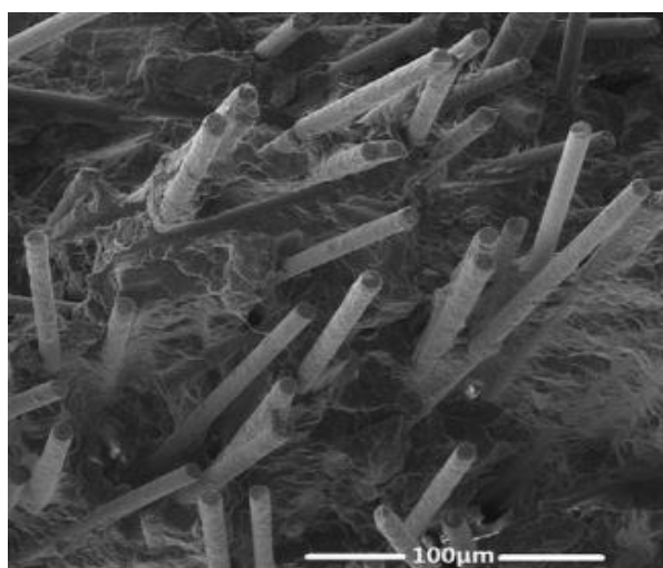
شکل ۲. تصویر SEM چندانسه پایه بسپاری حاوی الیاف کربن [۶۴].
