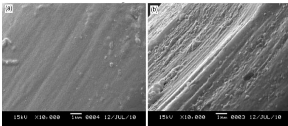
شکل ۵. بررسی سطح الیاف طبیعی رامی بعد از اصلاح به‌وسیله پلاسما فشار اتمسفری [۱۰۵].
