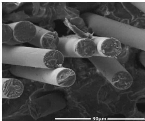
شکل ۲. تصویر SEM چندانسه پایه بسپاری حاوی الیاف کربن [۶۴].
