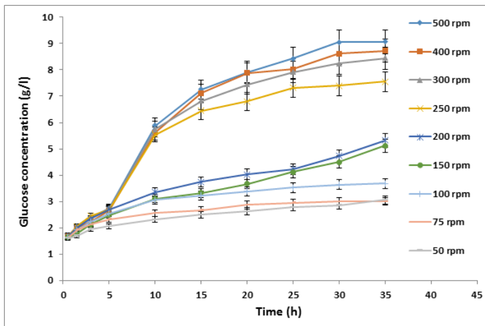
شکل ۲. گلوکز آزاد شده طی آزمایش‌های ۱ تا ۹ در دوره‌های مختلف همزن بین ۵۰ تا ۵۰۰ rpm و طی زمان. Figure 2. Glucose concentration at different stirring speeds ranging from 50 to 500 rpm versus time at experiments 1 to 9.
