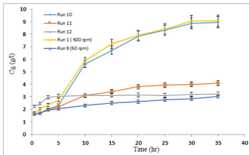
شکل ۷. مقدار گلوکز آزادشده در آزمایش‌های ۱۰ تا ۱۲ در مقایسه با آزمایش‌های ۱ و ۹.
