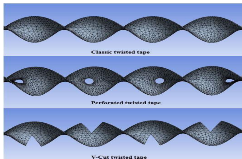
شکل ۷. مش‌بندی همزن‌های نواری پیچیده کلاسیک، حفره‌دار و V-Cut. Figure 7. Mesh of the classic, perforated, and V-Cut twisted tape mixer.
