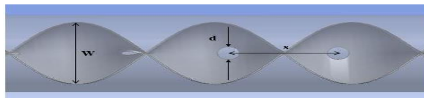
شکل ۳. ابعاد همزن نواری پیچیده حفره دار.
