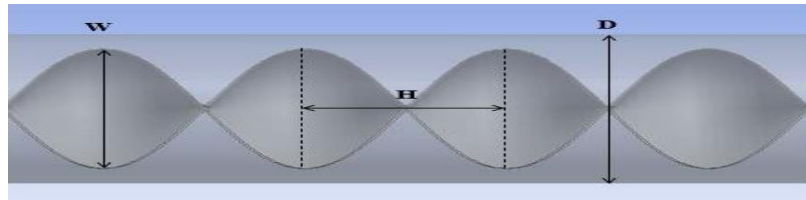
شکل ۱. ابعاد همزن نواری پیچیده کلاسیک.
