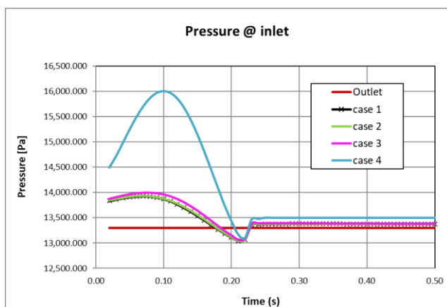
شکل ۱۱. فشار ورودی در یک دوره زمانی (تمامی حالت‌های گرفتگی).
