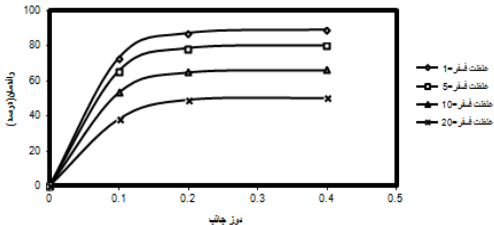
شکل ۴: تأثیر مقدار جاذب بر روی حذف فسفر معدنی با استفاده از نانولوله‌های کربنه چندجداره در زمان ۱۲۰ دقیقه، pH=7 ، در دمای 25^{\circ}C در غلظت 0.4 \text{ mg/L}
