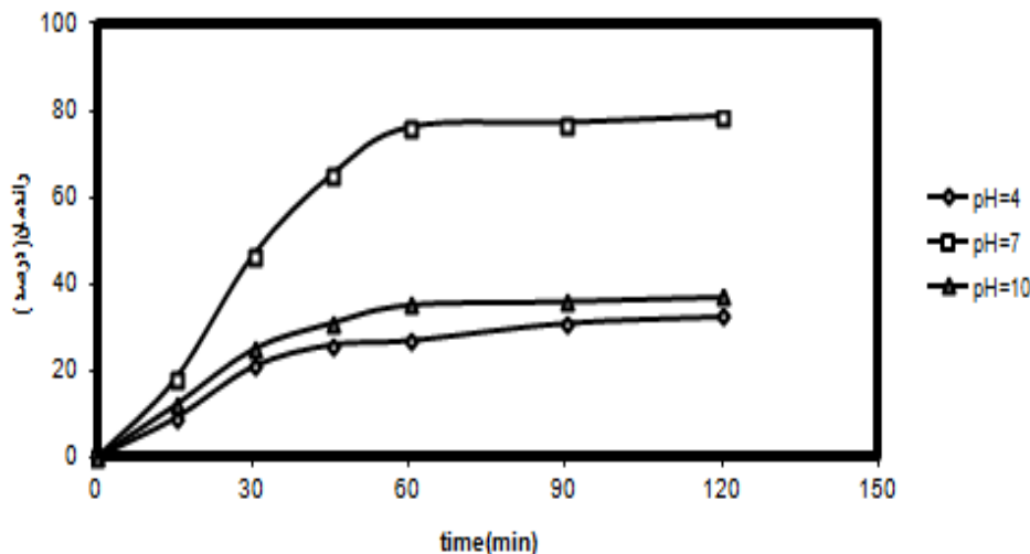
شکل ۳: تأثیر pH بر روی جذب فسفر با استفاده از نانولوله‌های کربنی چند جداره در زمان ۱۲۰، در دمای ۲۵ °C، در غلظت ۵mg/l ماده فسفر و غلظت ۰/۰۲g/L جاذب
