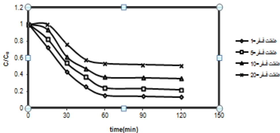
شکل ۵: تأثیر مقدار غلظت اولیه ماده فسفر معدنی بر روی حذف فسفر معدنی با استفاده از نانولوله‌های کربنی چندجداره در زمان ۱۲۰ دقیقه مختلف، pH=7 ، در دمای 25^{\circ}C و غلظت 0.4 \text{ mg/L} جاذب
