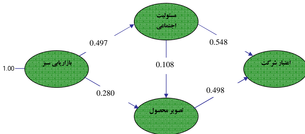
شکل 2. مدل برازش شده پژوهش در حالت استاندارد
