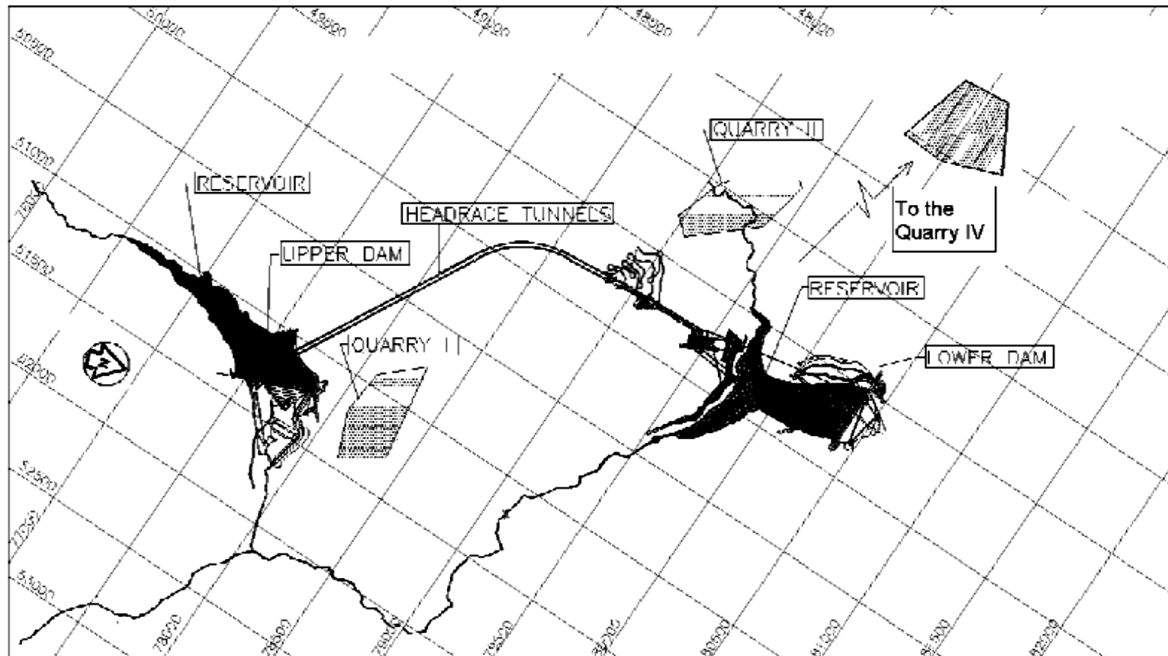
شکل ۱- شمای کلی پروژه ی تلمبه ذخیره ای سیاه بیشه
