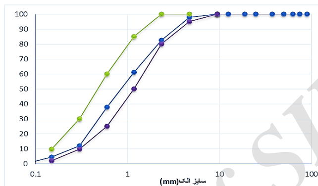
شکل 5- نمودار دانه بندی طرح 5
