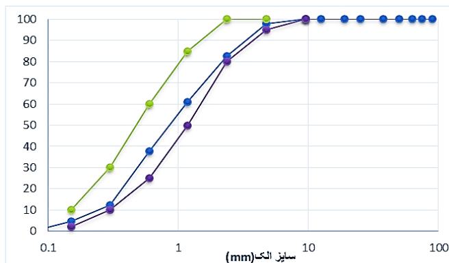
شکل 4- نمودار دانه بندی طرح 4
