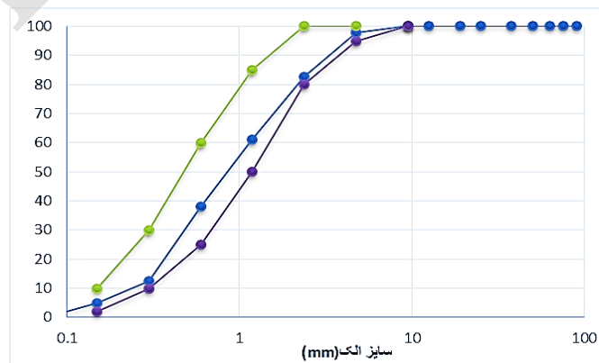
شکل 3- نمودار دانه بندی طرح 3
