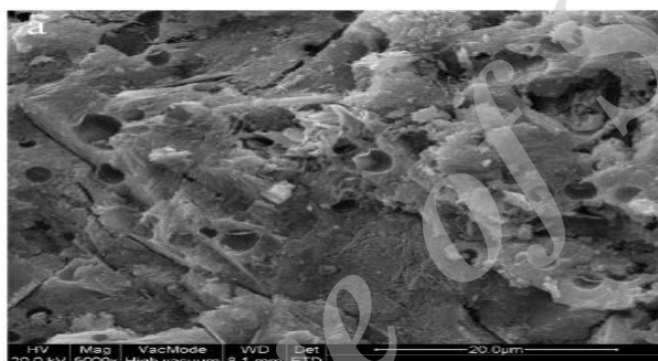
شکل 2 - تصویر SEM رسوب کلسیم کرنات در ماتریس بتن [36]
