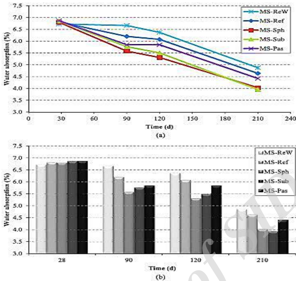
شکل 3- جذب آب نمونه های بتن با و بدون باکتریایی در معرض محیط سولفات در زمان های مختلف و سنین مختلف [39]
