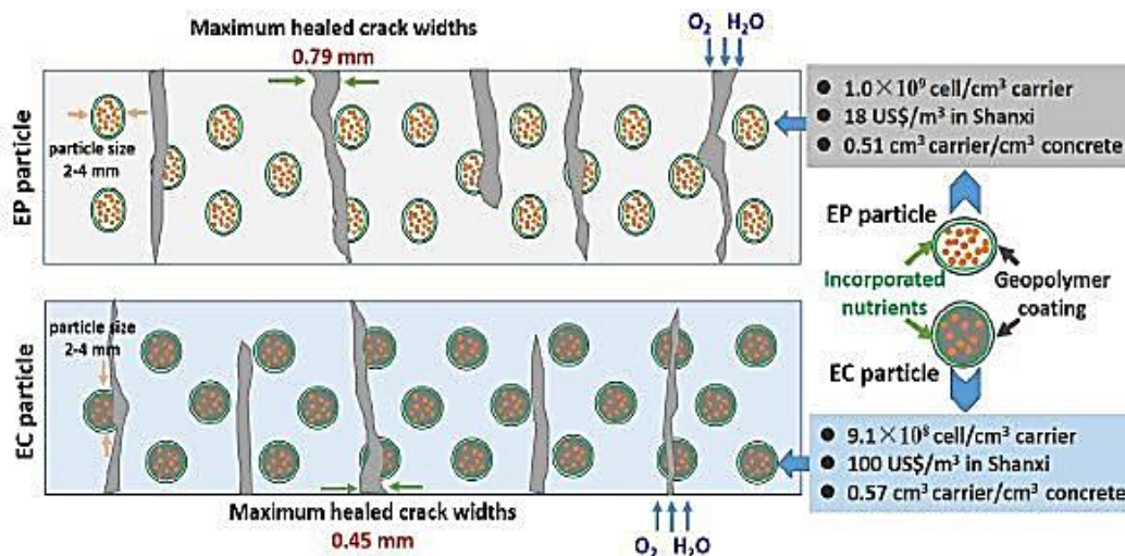
شکل 1 - عملکرد خودترمیمی با استفاده از روش امپولایزیشن باکتری ها [35]
