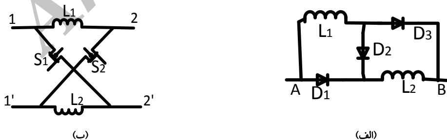
شکل ۲- واحد کلیدزنی سلفی (الف) کلیدزنی سلفی غیرفعال (ب) کلیدزنی سلفی فعال
