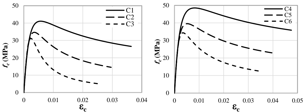
شکل ۴- روابط تنش- کرنش بدست آمده از نتایج تحلیل مدل های طراحی شده
