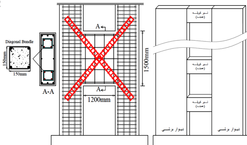
شکل ۱- جزئیات مقطع دیوار برشی کوبل شده
