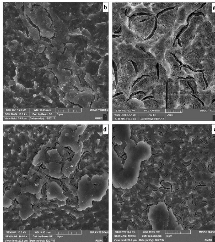
شکل ۴ - تصاویر FE-SEM از سطح تیتانیوم پوشش داده شده با (a) \text{TiO}_2(70\%)\text{-RuO}_2(30\%) ، (b) \text{TiO}_2(70\%)\text{-RuO}_2(25\%) ، (c) \text{TiO}_2(70\%)\text{-RuO}_2(20\%)\text{-SnO}_2(10\%) ، (d) \text{TiO}_2(70\%)\text{-RuO}_2(15\%)\text{-SnO}_2(15\%) ، \text{SnO}_2(5\%)
