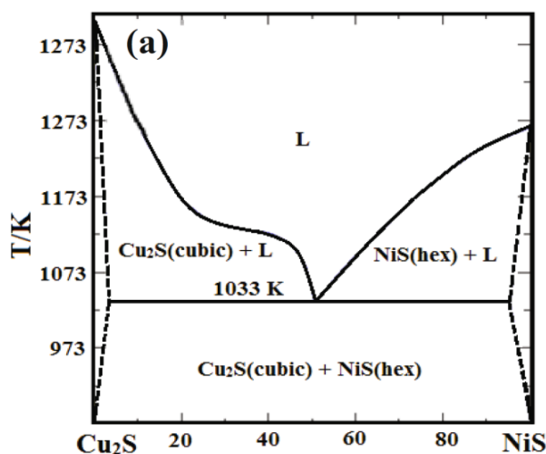
شکل ۱- نمودار فاز سیستم Cu_2S-NiS
