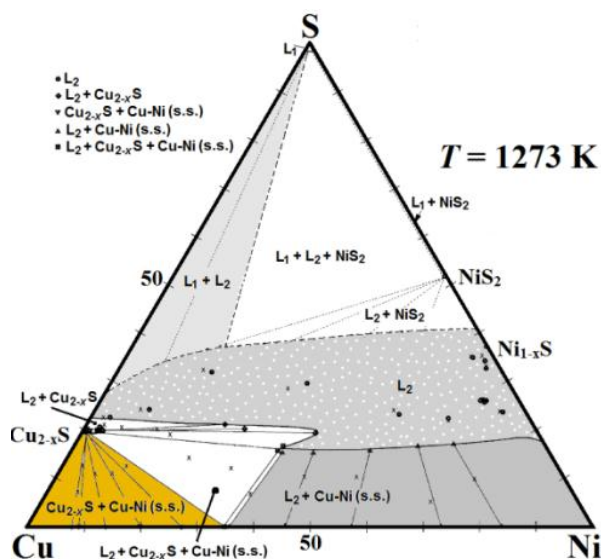
شکل ۲- نمودار فاز سیستم Cu-Ni-S در دمای ۱۲۷۳ درجه کلونین
