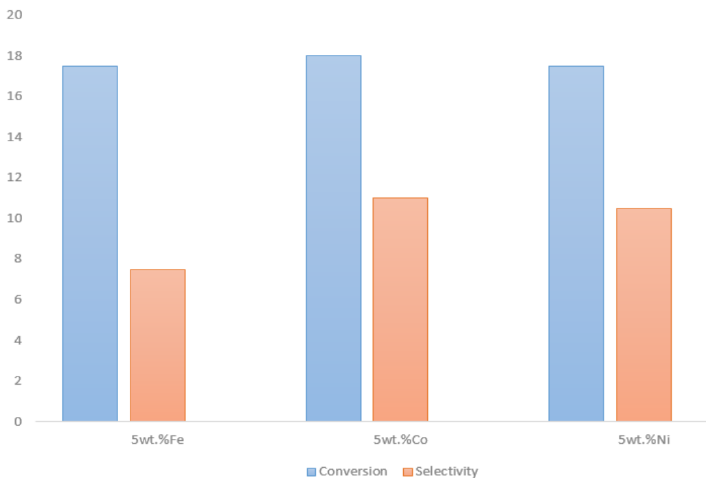
شکل ۲- اثر نوع فلز بر فعالیت و انتخاب‌پذیری C_2 از 5wt.\%XWO_4/2wt.\%Mn/SiO_2 در شرایط واکنش 800^\circ C درجه سانتی‌گراد و فشار 0.1 مگاپاسکال، 0.2 گرم کاتالیزور، ۵ ساعت.
