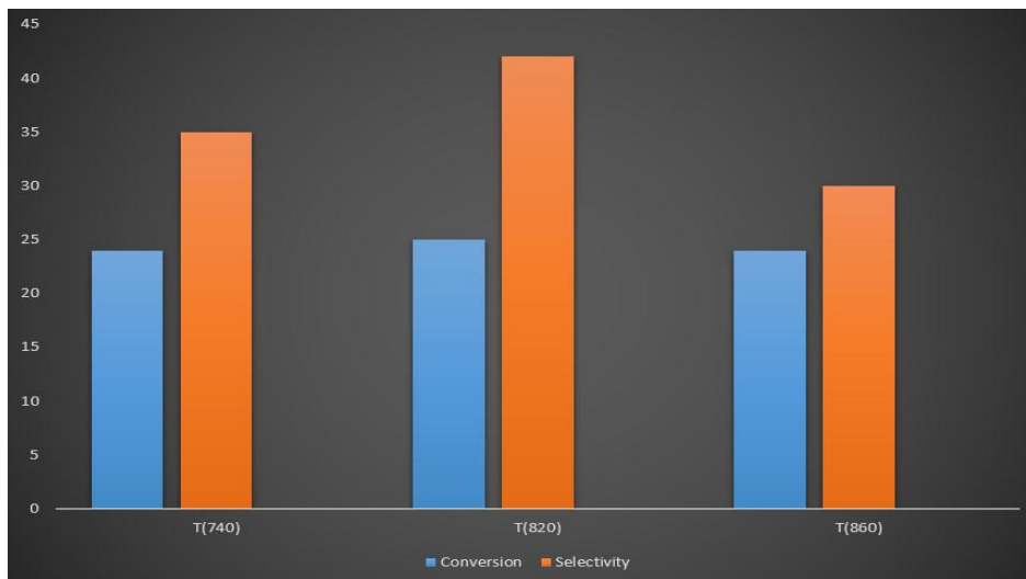
شکل ۴- اثر دمای واکنش (بر حسب درجه سانتی گراد) بر فعالیت و انتخاب پذیری C_2 از کاتالیزور MgO با استفاده از CH_4/O_2 = 4
