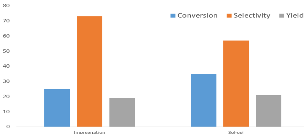
شکل ۳- اثر روش آماده سازی بر روی تبدیل، انتخاب پذیری C 2 و بازدهی در حضور کاتالیزور 5 wt.%Na 2 WO 4 /1.9 wt.%Mn/SiO 2 تهیه شده با روش های سل-ژل و تلقیح در شرایط واکنشی ۸۲۵ درجه سانتی گراد و نسبت متان به اکسیژن ۲/۵.
