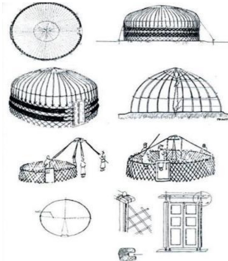
تصویر شماره ۱- نقشه و مراحل برپا کردن آلاجیق (URL3)
