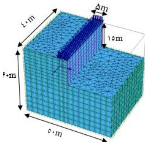
شکل (۱): مدل گودبرداری مورد بررسی
