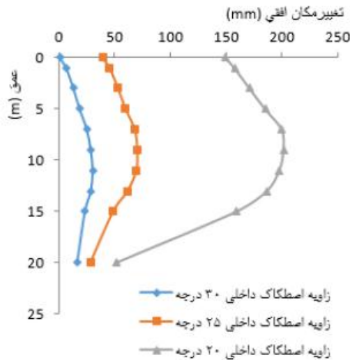
شکل (۴): نتایج تغییر مکان‌های افقی شمع کناری با زاویه اصطکاک داخلی ۲۰، ۲۵ و ۳۰ درجه و چسبندگی 20\text{ kPa}
