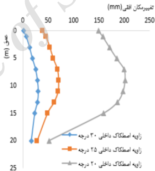
شکل (۵): نتایج تغییر مکان‌های افقی شمع میانی با زاویه اصطکاک داخلی ۲۰، ۲۵ و ۳۰ درجه و چسبندگی 30\text{ kPa}
