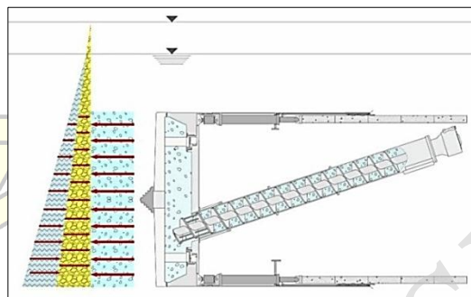
شکل ۸: تعادل فشار زمین [۵]
