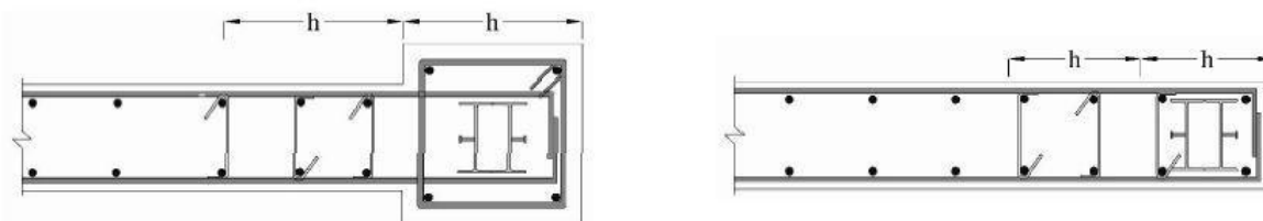
شکل ۳: جزئیات اجرایی فولاد عرضی در اجزاء مرزی.
