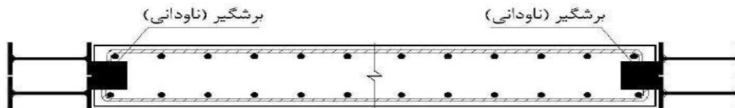
شکل ۱: ستون غیرمدفون در دیوار برشی.
