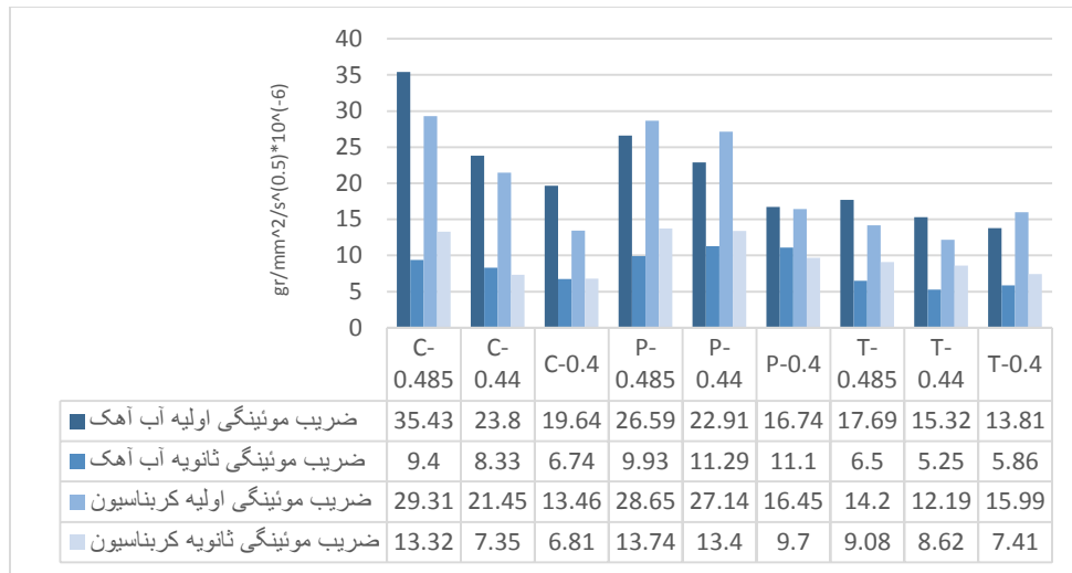
شکل ۶: مقایسه ضریب موئینگی اولیه و ثانویه ۱۱۹ روزه ملات‌های نگهداری شده در آب آهک و محیط کربن‌اسیون.
