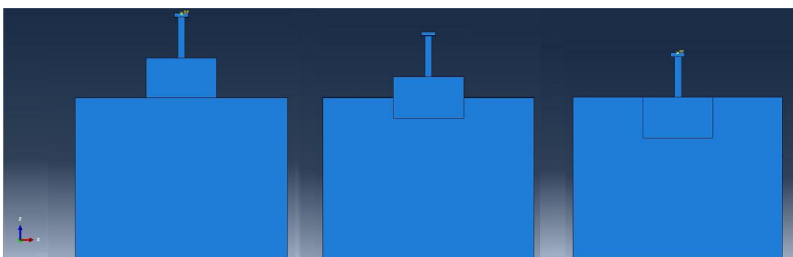
شکل ۴: حالت‌های مختلف مدفون شدگی فونداسیون در سیستم اندرکنشی D=10 و D=5 و D=0 متر.
