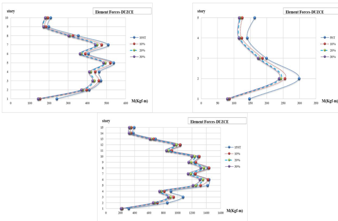
شکل ۱۳: نیروی داخلی ستون مدل ۵، ۱۰ و ۱۵ طبقه تحت رکورد Duzce.
