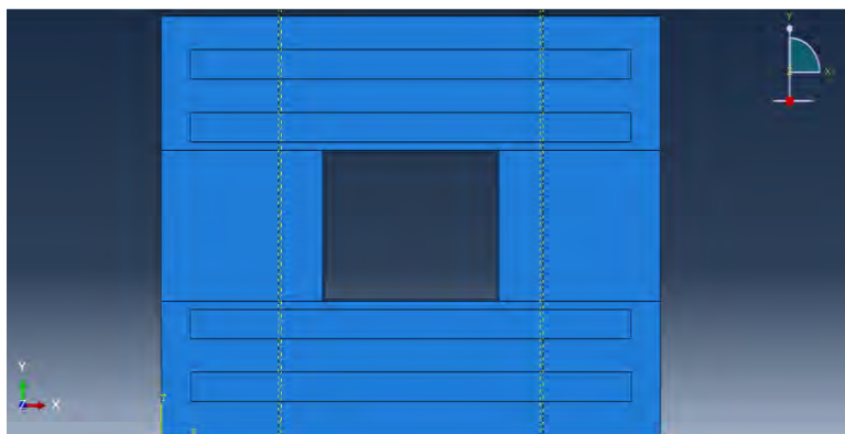
شکل ۳: مدل سازی دال بتنی مسلح شده.
