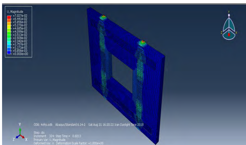
شکل ۳۱: حداکثر تغییر مکان (تمام شکل (m)) نمونه BOX-2
