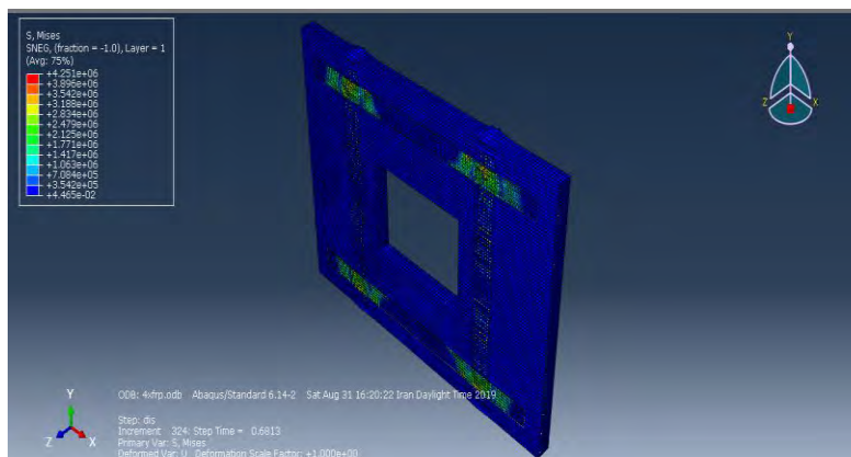
شکل ۳۰: تنش ون میسز (تمامی شکل (pa)) نمونه BOX-2
