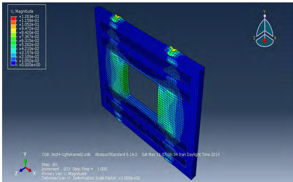
شکل ۱۳: حداکثر تغییر مکان (تمامی شکل (m)) نمونه 2- GFRP
