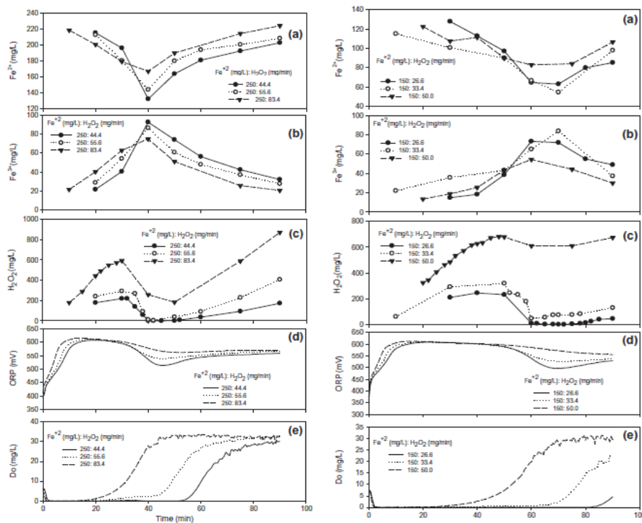
شکل ۴: تغییرات یون آهن ۲ و ۳، آب اکسیژنه، ORP و DO در نسبت‌های مختلف Fe/H_2O_2 در تزریق تدریجی آب اکسیژنه
