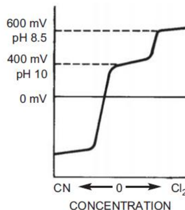
شکل ۳: نمودار تغییرات ORP در حین واکنش تخریب سیانید
