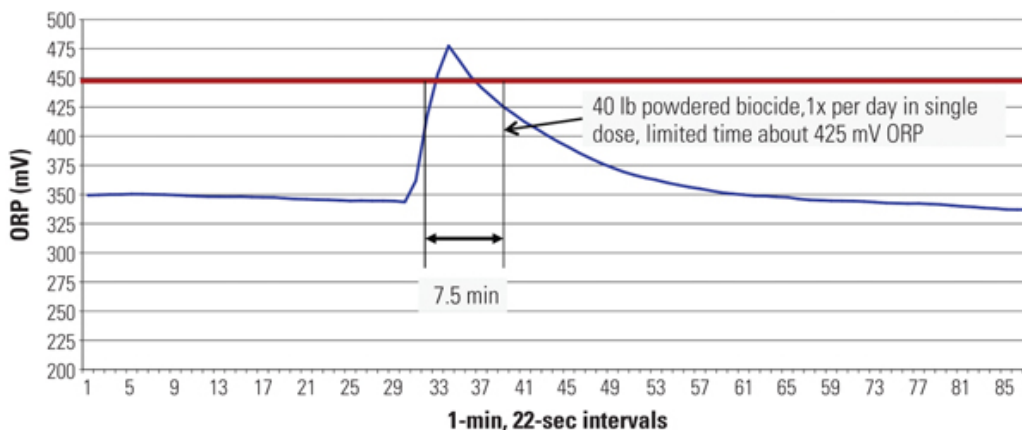
شکل ۶: تغییرات مقدار ORP بعد از وارد نمودن گندزدا
