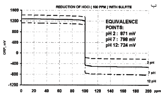
شکل ۲: رصد واکنش اکسایش و کاهش (الف) غیروابسته به pH و (ب) وابسته به pH
