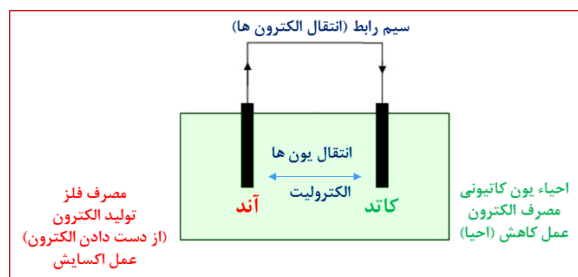
شکل ۱: شماتیک یک پیل الکتروشیمیایی
