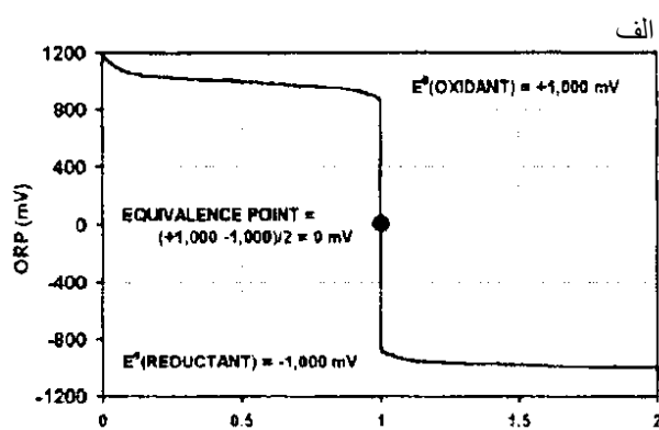
شکل ۲: رصد واکنش اکسایش و کاهش (الف) غیروابسته به pH و (ب) وابسته به pH
