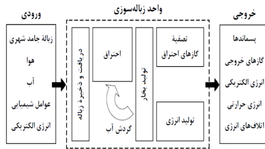
شکل ۲- فرآیندها، ورودی و خروجی برای یک واحد زباله‌سوز (شفیعی، ۱۳۹۴)
