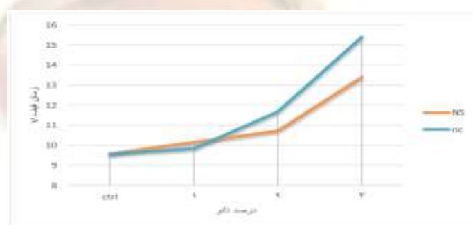
نمودار ۲؛ تاثیر میزان استفاده از نانوسیلیس و نانو مس بر زمان قیف V
