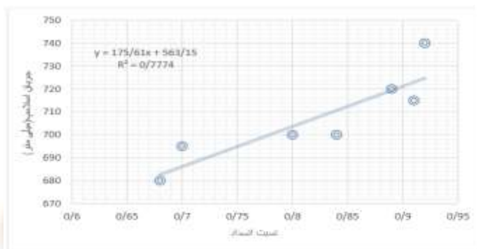
نمودار ۵: بررسی ارتباط بین نسبت انسداد و جریان اسلامپ در مخلوط های حاوی ذرات نانو
