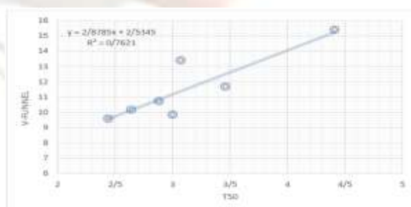
نمودار ۴؛ ارتباط بین زمان قیف V و T ۵۰ در مخلوط‌های با درصد‌های مختلف نانو
