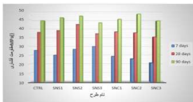
نمودار ۶؛ تغییرات مقاومت فشاری در درصد‌های متفاوت جایگزینی نانوسیلیس و نانومس
