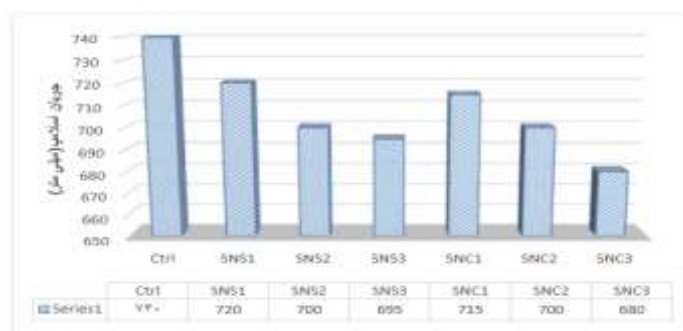
نمودار ۱؛ آزمایش جریان اسلامپ در درصدهای متفاوت نانو
