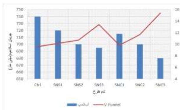
نمودار ۳؛ بررسی همزمان نتایج جریان اسلامپ و قیف V در مخلوط‌های با درصد‌های مختلف نانو
