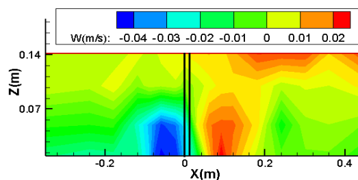
الف) نتایج آزمایشگاهی آبشکن دو ردیفه در امتداد هم A. Experimental results of parallel groyned
