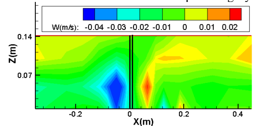
ج) نتایج آزمایشگاهی آبشکن دو ردیفه زیگزاگی C. Experimental results of Zigzag groyned
