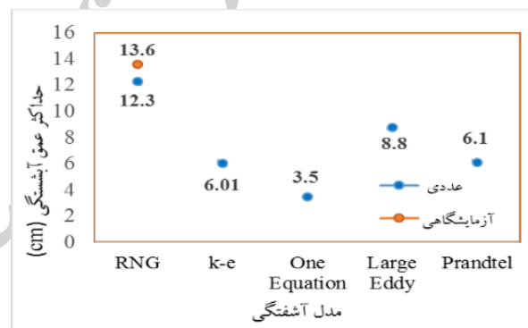
شکل ۳- مقایسه حداکثر عمق آبشستگی حاصله از مدل‌های مختلف آشفتگی
