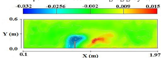
د) نتایج شبیه‌سازی عددی آبشکن دو ردیفه زیگزاگی d. Numerical results of Zigzag groyne
