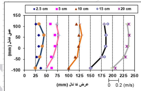
مقطع X = 0
