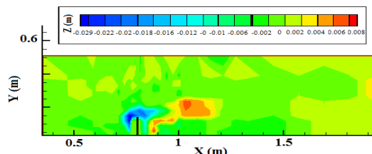
الف) نتایج آزمایشگاهی آبشکن دو ردیفه در امتداد هم a. Experimental results of parallel groyne
