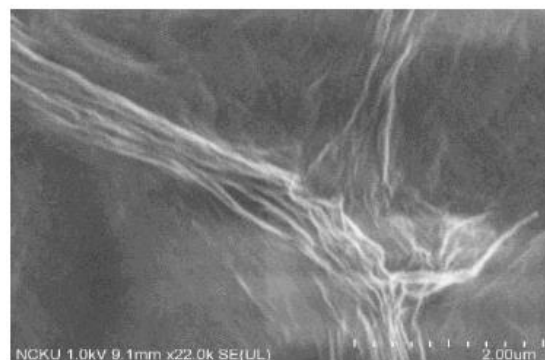
شکل ۳- تصویر FE-SEM گرافن اکسید عامل دار (GO-GAA) Fig. 3 FESEM of GAA-GO
