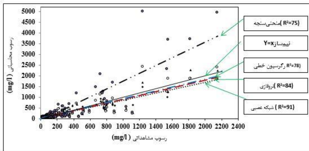
شکل ۳- نمودار پراکنش نتایج مدل‌های شبکه عصبی مصنوعی، سیستم نروفازی، رگرسیون خطی و منحنی سنجه
