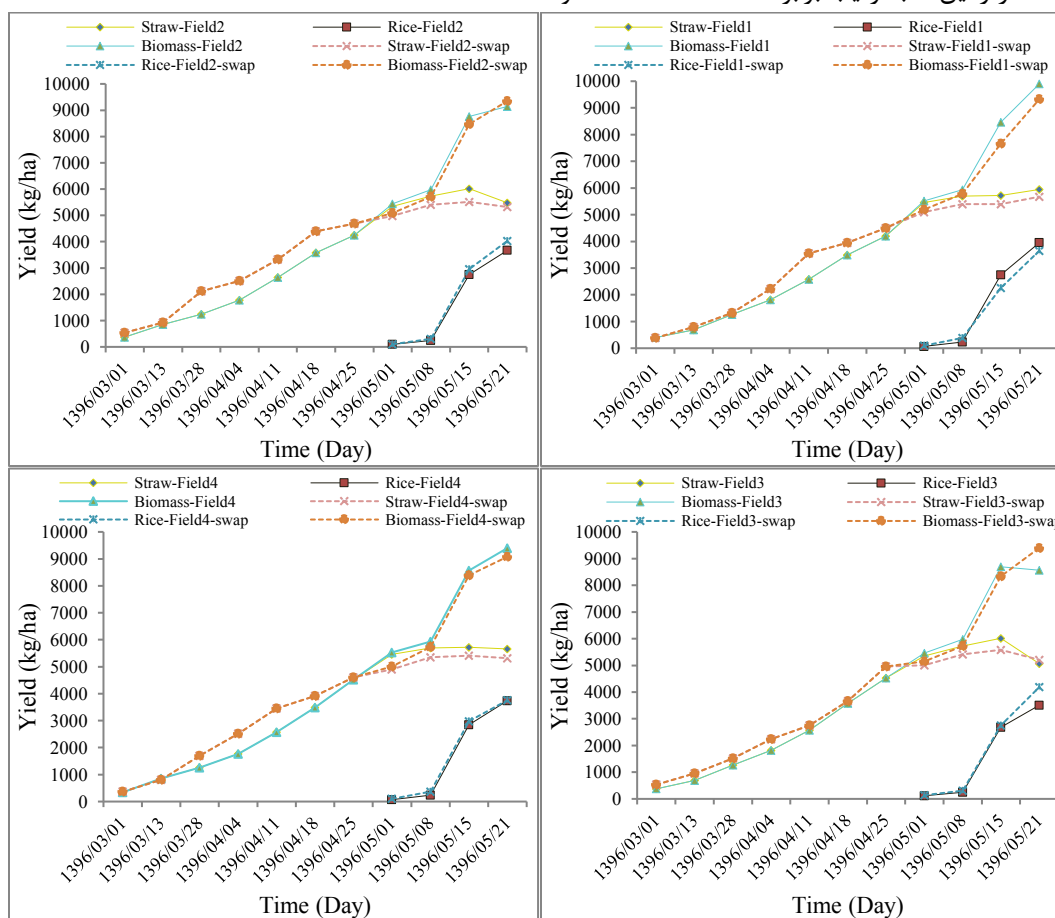
شکل ۲- عملکرد اندازه‌گیری شده و شبیه‌سازی شده شلتوک، کاه و زیست‌توده گیاه برنج Fig. 2 Measured and simulated yield of paddy, straw and biomass of rice plant with
