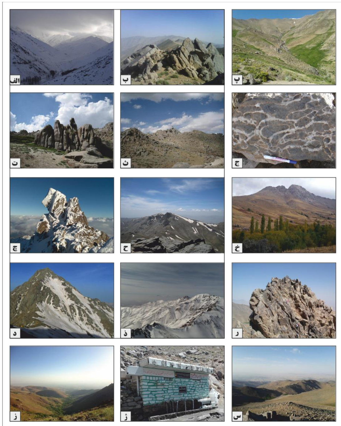
شکل ۴. نماهایی از: الف: قله کمرلرزان، ب: چهارقله، پ: دامنه‌های قله یخچال صاحب‌الزمان، ت و ث: کلاه‌قاسی، ج: واحد تداخلی میان گرانیب و گابرو در مسیر بین قله‌های کلاغ‌لان و کوه دائم‌برف، چ: قله الوند، ح: آلموقولا، خ: کرکس، د: قزل‌ارسلان، ذ: دائم‌برف، ر: کلاغ‌لان، ز: دورنمای دوزخ‌دره، ژ: یکی از چشمه‌های تاریک‌دره و س: دورنمای تاریک‌دره از ارتفاعات مشرف بر آن (شکل ج از رشید، ۱۳۸۸ و چ از علی بیات (وبسایت هیئت کوهنوردی و صعودهای ورزشی استان همدان) اخذ شده است).
