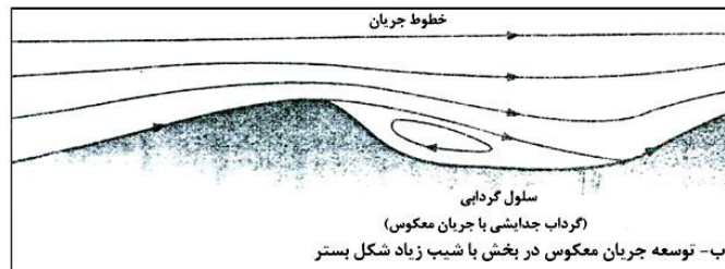
شکل ۴. خطوط جریانی بر روی اشکال بستر. الف- فرسایش در بخش فرورفته در اثر جریان. ب- توسعه جریان‌های گردابی (معکوس) در بخش با شیب زیاد (نیکولز، ۲۰۰۹)
