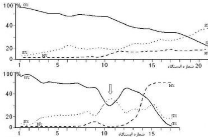
شکل ۱۰. روند ریزشوندگی دانه‌های در اندازه گراول بدون ناپیوستگی (بالا) در رودخانه قفل‌رود تویسرکان و با ناپیوستگی رسوبی (پایین) در رودخانه سیمینه‌رود (خدابخش، ۱۳۹۳). علامت پیکان نشان‌دهنده محل پیوستن شاخه فرعی صالح‌آباد به سیمینه‌رود است. S, G و M به ترتیب نشان‌دهنده دانه‌های در اندازه گراول، ماسه و گل است.
