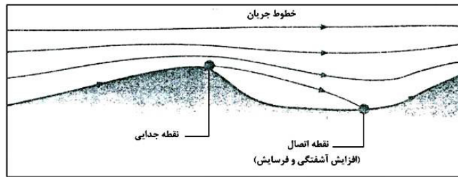
الف- فرسایش در بخش فرورفته شکل بستر
