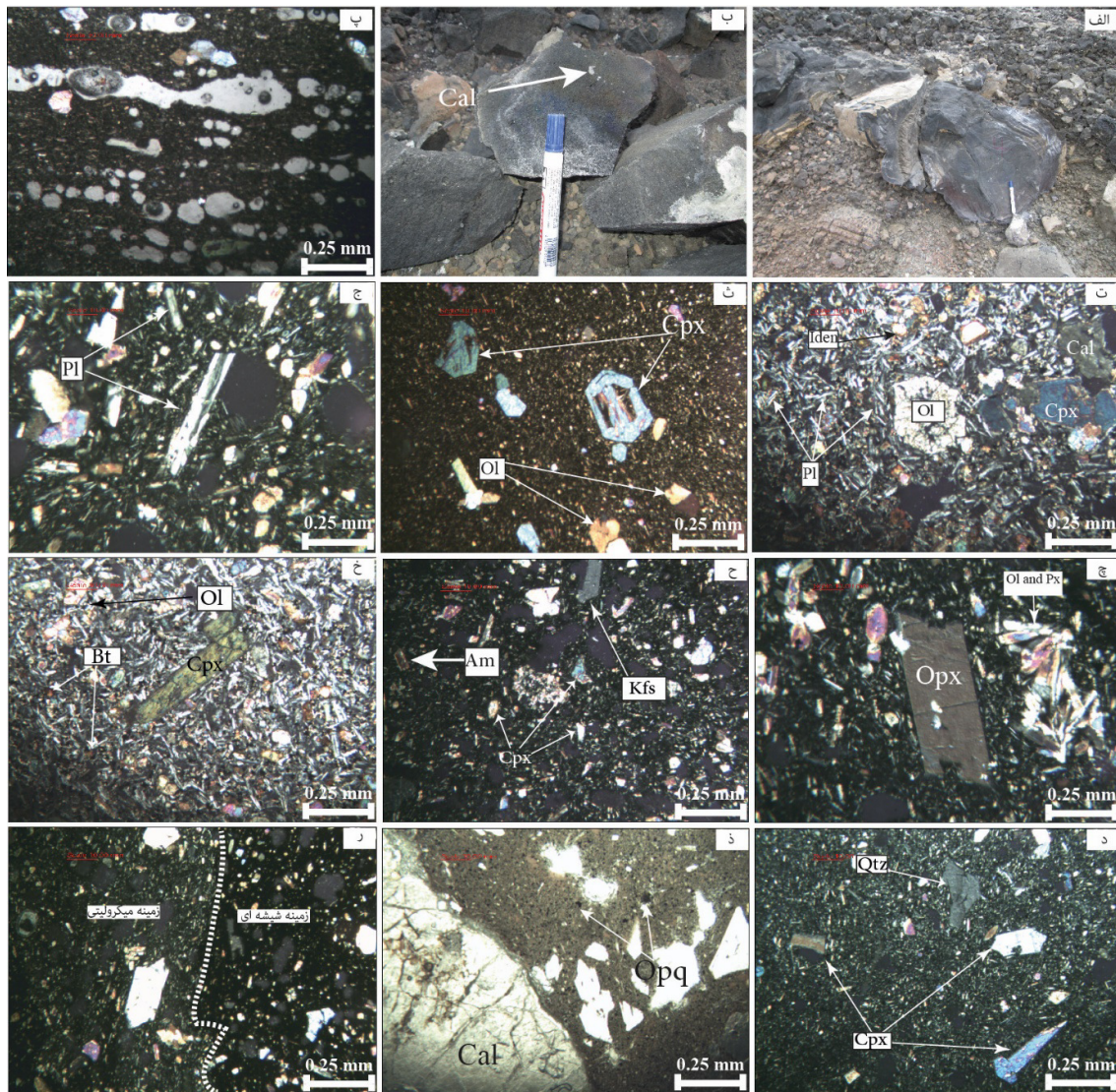
شکل ۶: الف: نمونه صحرایی سنگ‌های بازالتی منطقه کوه‌سیاه و طهمورت. ب: نمونه دستی سنگ بازالتی پ: تصویر میکروسکوپی از سنگ بازالتی که در حالت XPL گرفته شده است. ت: نمونه‌ای از بلورهای اولیوین با حاشیه ایدینسیتی شده حالت XPL، ت: کلینوپیروکسن در یک زمینه شیشه‌ای حالت XPL، ج: بلورهای پلاژیوکلاز با ماکل پلی‌سنتتیک حالت XPL، ج: اورتوپیروکسن در یک زمینه شیشه‌ای حالت XPL، ح: بلورهای ریز آمفیبول همراه با فلدسپار پتاسیم حالت XPL، خ: نمونه‌ای از بلورهای ریز بیوتیت حالت XPL، د: نمونه‌ای از بلور کوارتز اولیه دارای حاشیه واکنشی حالت XPL، ذ: نمونه‌های میکروسکوپی از کانی‌های اوپک و کلسیت‌های ثانویه حالت PPL، ر: زمینه‌ی شیشه‌ای و میکرولیتی در سنگ‌های ناحیه مورد مطالعه حالت XPL، علائم اختصاری کانی‌ها بر روی شکل از (کرتز، ۱۹۸۳).
