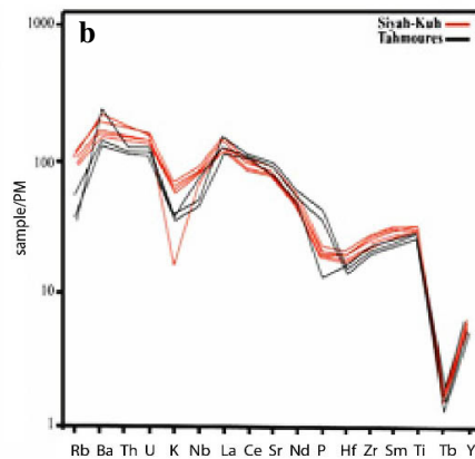
شکل ۹. a الگوی REE نرمالیزه به کندریت (مقادیر از ناکامورا، ۱۹۷۴). b نمودار عنکبوتی نرمالیزه شده به گوشته‌ی اولیه (مقادیر از مک دوناف و همکاران، ۱۹۹۲)
