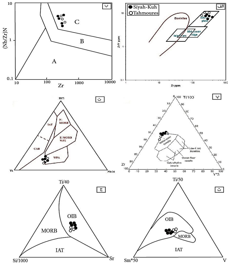
شکل ۱۳. الف: نمودار Zr در مقابل Zr/Y (پیرس و نوری، ۱۹۷۹) ب: نمودار ارائه شده توسط تیلیمونت و تگیه (۱۹۹۴) که در آن محدوده A معرف زون فرورانشی، B زون برخوردی و C سنگ‌های آکالن درون صفحه‌ای است پ: نمودار مثلثی Ti/100-Zr-Y*3 (پیرس و کان، ۱۹۷۳) ت: نمودار مثلثی Hf/3-Th-Nb/16 (وود، ۱۹۸۰) که در آن IAT بیانگر تولیت-های جزایر قوسی و WPA بیانگر محیط درون صفحه‌ای و CAB بیانگر بازالت‌های مرتبط با قوس قاره‌ای می‌باشد ث و ج: نمودار مثلثی Ti/40-Si/1000-Sr (ورمیش، ۲۰۰۶) که در آن (OIB) بیانگر بازالت‌های جزایر اقیانوسی، (IAB) بیانگر بازالت‌های جزایر قوسی و (MORB) بیانگر بازالت‌های پشته‌های میان‌اقیانوسی می‌باشد.
