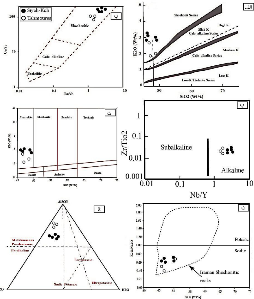
شکل ۸. الف: نمودار در مقابل SiO 2 K 2 O (پسریلو و تیلور، ۱۹۷۶). ب: نمودار Ta/Yb در مقابل Ce/Yb (پیرس، ۱۹۸۲). پ: نمودار Nb/Y در مقابل Zr/TiO 2 (وسکوئز و آلتنبرگر، ۲۰۰۵). ت: نمودار SiO 2 در مقابل K 2 O برای طبقه‌بندی شوشونیت‌ها (مکنزی و چاپل، ۱۹۷۲). ث: نمودار SiO 2 در مقابل K 2 O/Na 2 O جهت تعیین سدیک و پتاسیک بودن شوشونیت‌ها که نمونه‌های مورد مطالعه در محدوده‌ی سدیک قرار گرفته‌اند (آفتابی و عطاپور، ۲۰۰۰)
