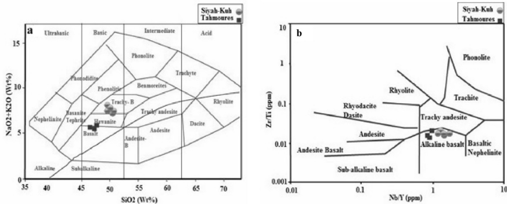
شکل ۷. نمودار طبقه‌بندی SiO 2 در مقابل Na 2 O+K 2 O از (کاکس و همکاران، ۱۹۷۹). b: نمودار طبقه‌بندی Nb/Y در مقابل Zr/Ti و e: نمودار طبقه‌بندی Nb/Y در مقابل SiO 2 از (وینچستر و فلوید، ۱۹۷۷)
