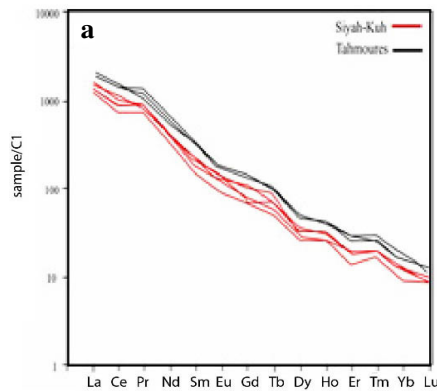
شکل ۹. a الگوی REE نرمالیزه به کندریت (مقادیر از ناکامورا، ۱۹۷۴). b نمودار عنکبوتی نرمالیزه شده به گوشته‌ی اولیه (مقادیر از مک دوناف و همکاران، ۱۹۹۲)
