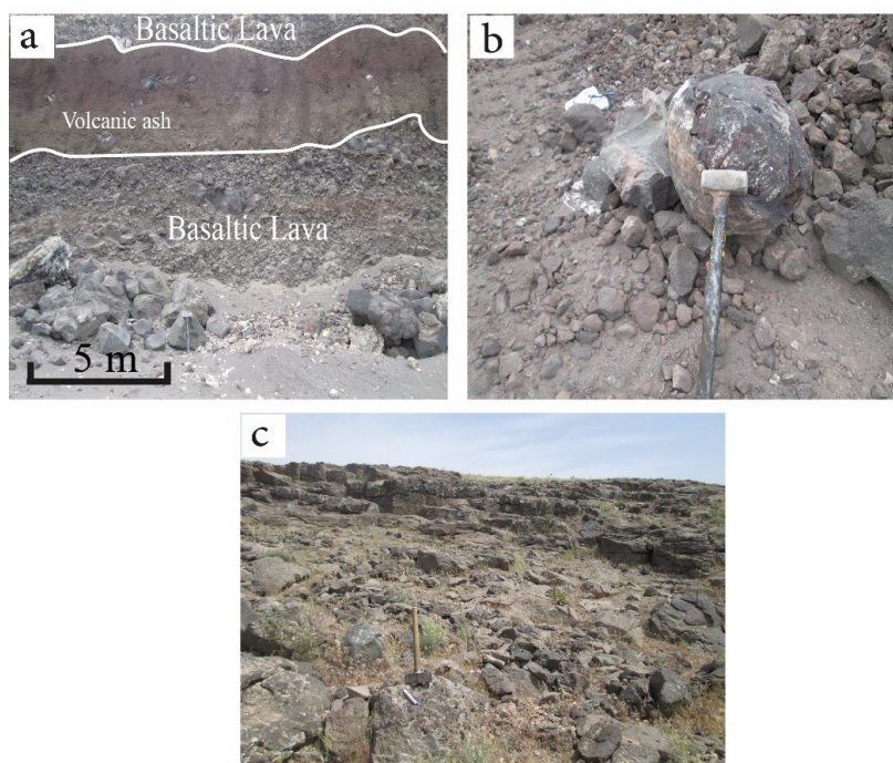
شکل ۵. a: تناوبی از لایه‌های گدازه و خاکستر در آتشفشان کوه سیاه (دید به سمت غرب) b: نمایی از بمب‌های آتشفشانی دوکی شکل در آتشفشان کوه سیاه c: سنگ‌واریزه‌های بازالتی (دید به سمت شرق)
