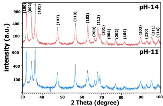
شکل (۲): الگوی پراش پرتو ایکس ساختار ZnO در pH های ۱۱ و ۱۴.
