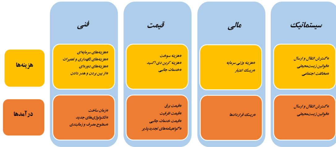
شکل ۳ مسئله ریسک مؤثر در محاسبه جریان پول نقد شرکت
