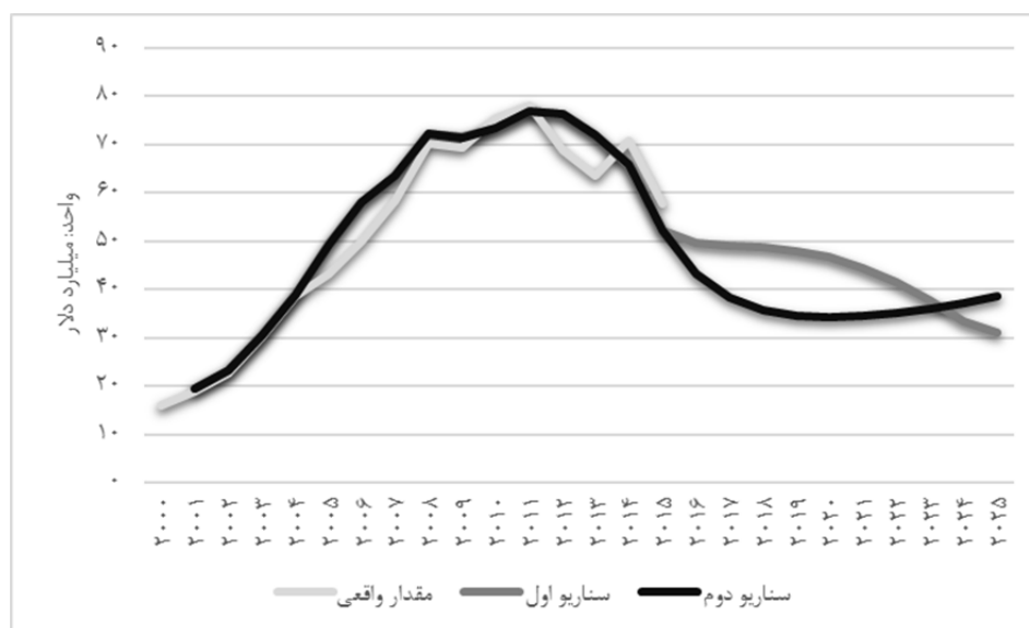
نمودار ۱۴. پیش بینی واردات کل ایران طی افق ۱۴۰۴ (بازه زمانی ۲۰۲۵)
