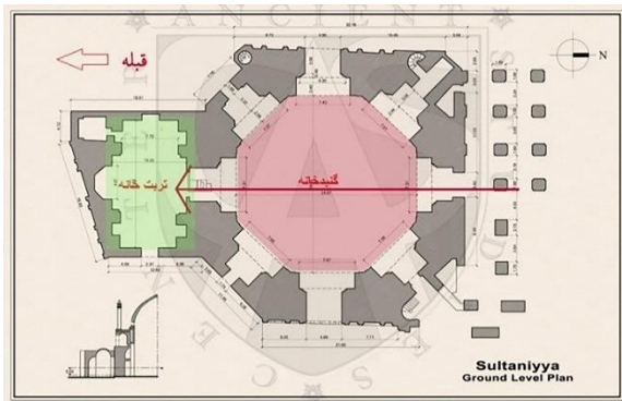
تصویر ۱۱: پلان مقبره الجایتو (گنبد سلطانیه) که نحوه جانمایی گنبدخانه و تربت خانه و همچنین نحوه حرکت در فضا و رسیدن به مزار را نشان می دهد. Fig. 11: The plan of the Al-Jaytuo (Soltanieh Dome), which depicts how to locate the dome and the Torbat-Khaneh, as well as how to move in and reach the tomb.
