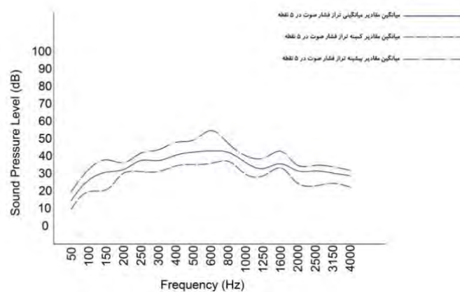
تصویر ۷: کمینه، میانگین و بیشینه تراز فشار صوت در سرا میرزا محمد (سرای کوچک) Fig. 7: Minimum, Average and Maximum SPL in Mirza Mohammad Sarâ (The small Sarâ)
