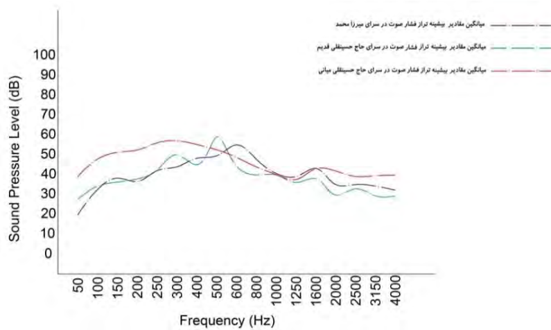
تصویر ۱۲: گراف‌های میانگین مقادیر بیشینه تراز فشار صوت در سه سرا
