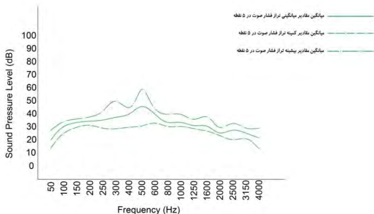
تصویر ۸: کمینه، میانگین و بیشینه تراز فشار صوت در سرای حاج حسین قدیم (سرای میانه)
