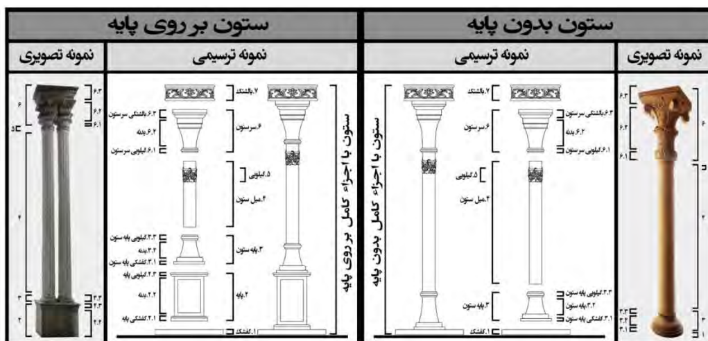
شکل ۶. معرفی تصویری اجزاء ستون در دو گونه اصلی: ستون بدون پایه (سمت راست) با نمونه تصویری خانه مصطفوی و ستون روی پایه (سمت چپ) با نمونه تصویری عمارت باغ گلشن (عقیف آباد).
