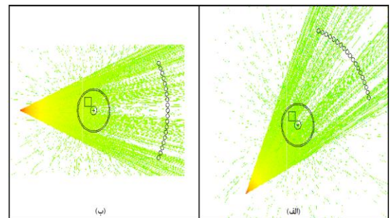
شکل ۳- ترابرد فوتون های پرتوی گامای چشمه تا آشکارساز با عبور از فانتوم. الف) زاویه ۴۵ درجه، ب) زاویه ۰ درجه
