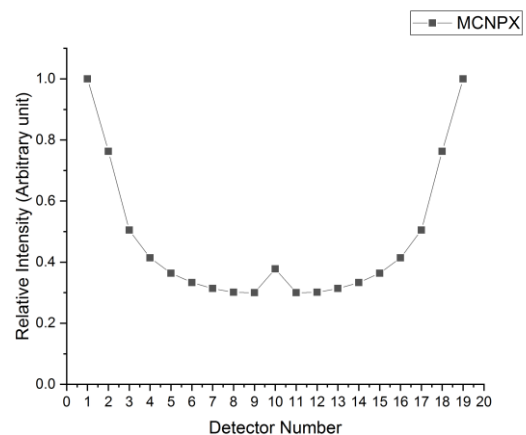
شکل ۶- پروجکشن روی زاویه صفر درجه برای فانتوم استاندارد صنعتی
