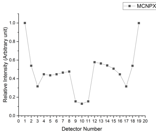
شکل ۷- پروجکشن روی زاویه صفر درجه برای فانتوم آزمون طراحی شده برای این پژوهش
