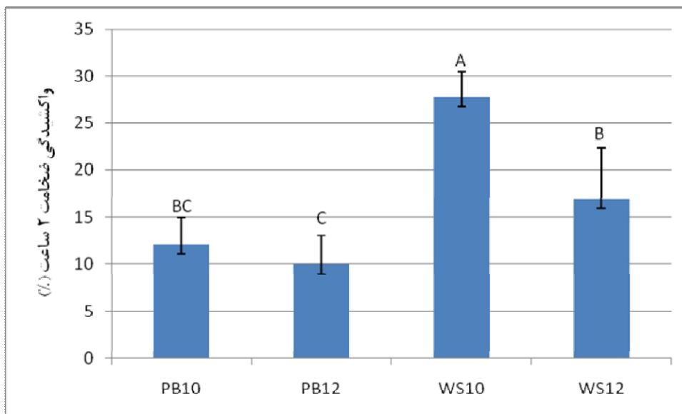
شکل 3. اثر نوع ماده لیگنوسولوزی و درصد چسب بر واکسیدگی ضخامت 2 ساعت
