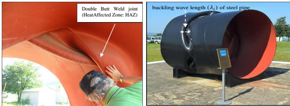
شکل ۱. پانچینگ در محل تقاطع لوله با گسل (کایا ۲۰۱۷) - زلزله ۱۹۹۹ کوکائیلی با جابجایی جانبی ۳ متر [۶]
