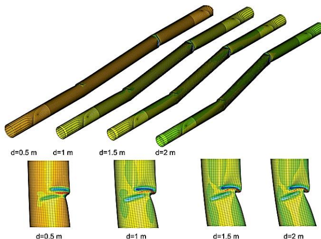
شکل ۲. کمانش موضعی در ناحیه فشاری [۴]
