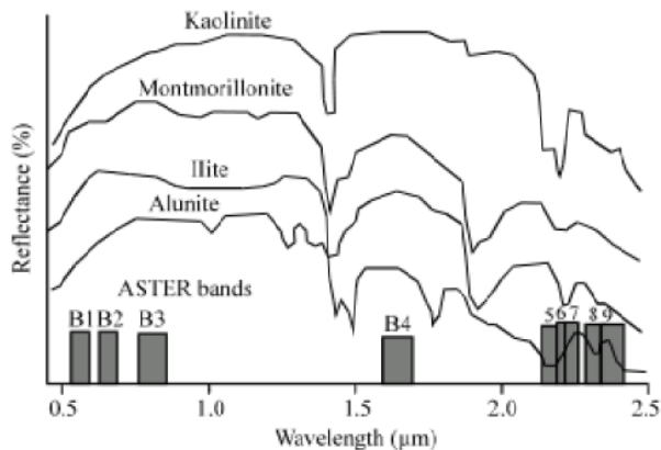
شکل ۲. کائولینیت، مونت‌موریلونیت، ایلیت، آلونیت و موقعیت باندهای استر [۴]
