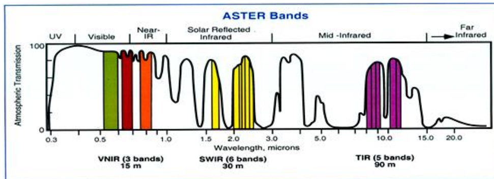
شکل ۱. محدوده باندهای سنجنده استر در طیف الکترومغناطیس [۳]
