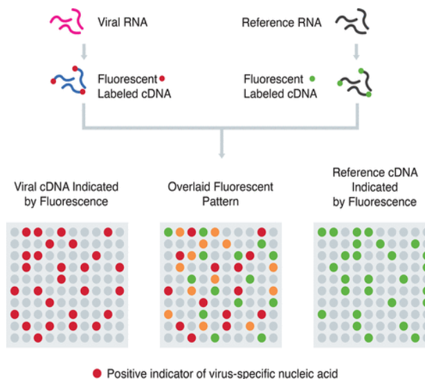
تصویر ۵. هیبریدیزاسیون نوکلئیک اسید با استفاده از ریز آرایه. cDNA ویروسی و cDNA رفرنس با استفاده از لیبل های فلئورسنت مختلف ترکیب شده و در داخل چاهک های ریز آرایه پوشانده شده با پروب های خاص DNA قرار می گیرند [۱۰].
