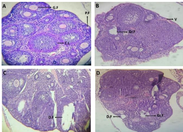
شکل ۴: میکروگراف برش عرضی از تخمدان کنترل (A) و تخمدان تجربی با داروی لورازپام در ۱۵ روز (B, C) و (بزرگنمایی \times 40 ). P.F: فولیکول اولیه، C.L: جسم زرد، G.F: فولیکول در حال رشد، Gr.F: فولیکول گرافت تخریب شده، V: رگ خونی، D.F: فولیکول در حال تخریب
