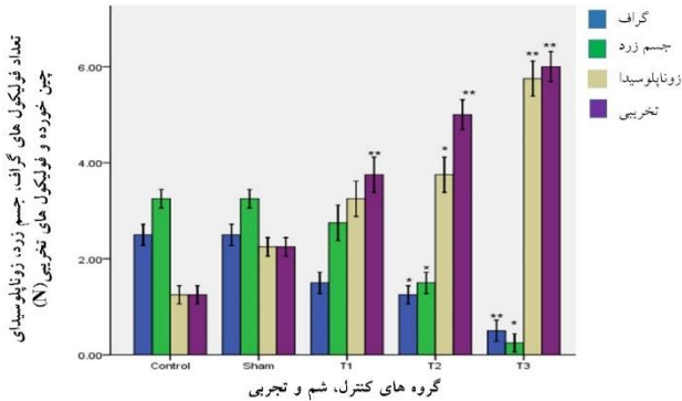
نمودار ۳: مقایسه تعداد فولیکول های گراف، جسم زرد، زوناپلوسیدای چین خورده و تخریبی در نمونه های کنترل، شم و تجربی. P < 0.05 و P < 0.001
